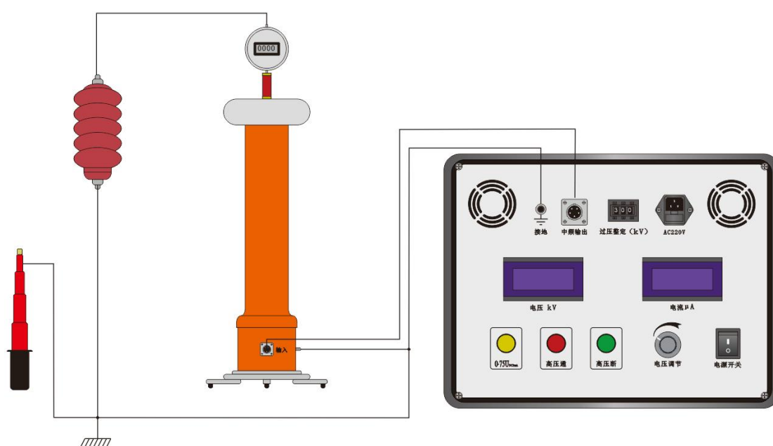
图 4 试验回路连接图
