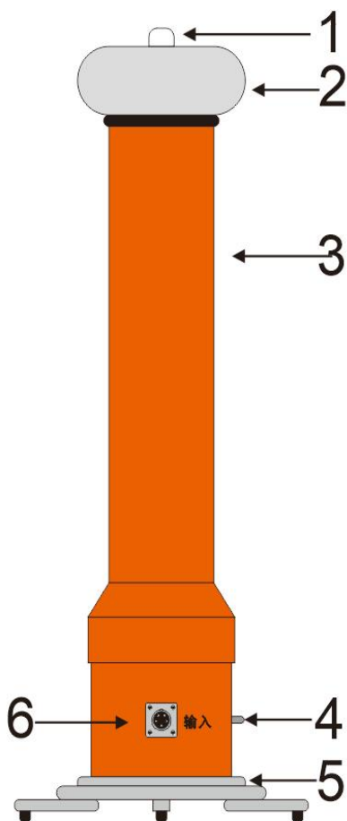
图 3 倍压筒示意图
