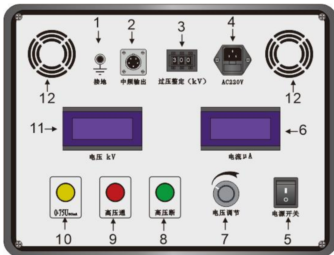
图2 面板布局图
